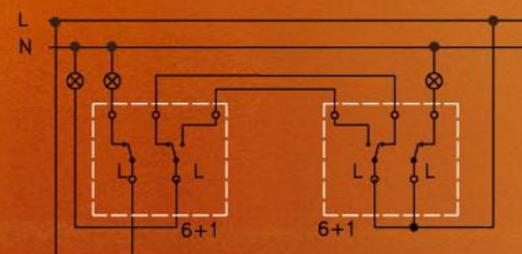
Zapojenie dvoch dvojpólových spínačov 6+1 (5A) a 6+1 (5A)
