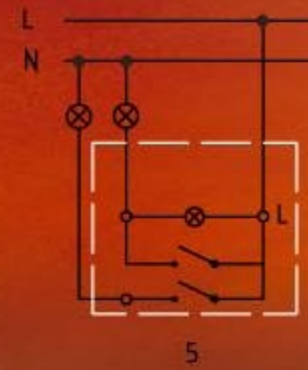
Sériový prepínač s podsvietením
